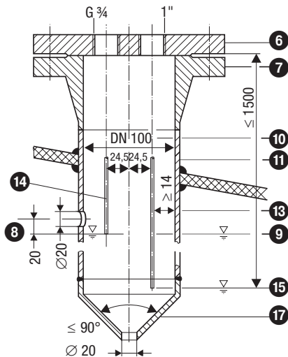
Fig. 6 Tubo di calma di protezione (da prevedere sul posto) per installazione all'interno della caldaia previsto per montaggio di un secondo apparecchio GESTRA
