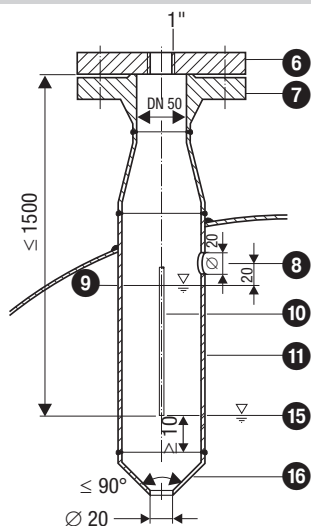
Fig. 5 Tubo di calma di protezione (da prevedere sul posto) per installazione all'interno della caldaia
