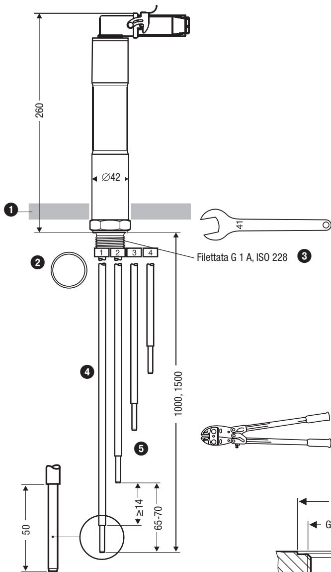
Fig. 2 NRG 1..-52 con connettore a cinque poli
