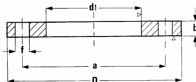
TIPO 01A
