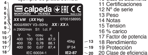
Ejemplo de placa bomba
